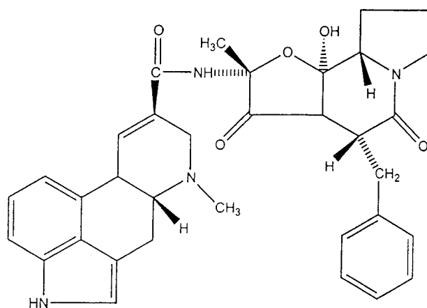
FIG. 3. Ergotamine.
