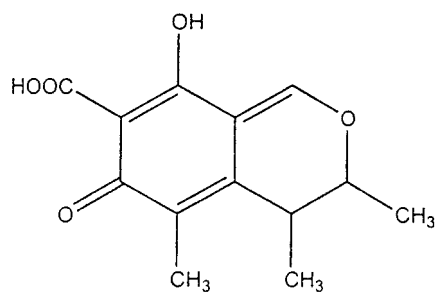
FIG. 2. Citrinin.
