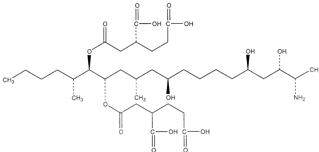
FIG. 4. Fumonisin B 1 .
