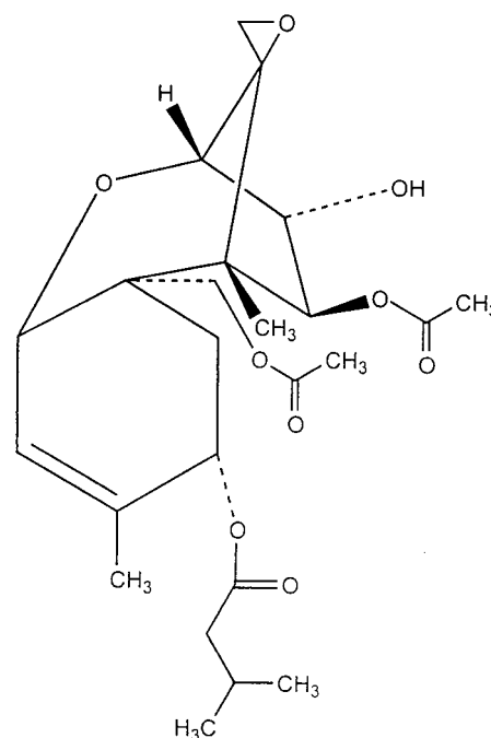
FIG. 7. T-2 toxin.
