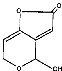
FIG. 6. Patulin.
