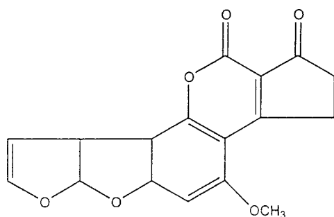
FIG. 1. Aflatoxin B 1 .
